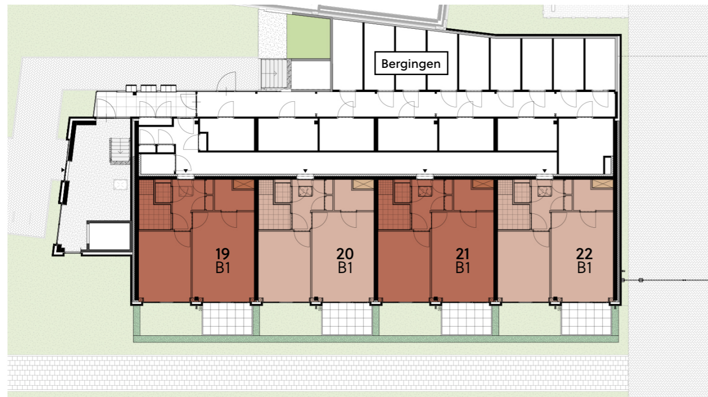
Begane grond
